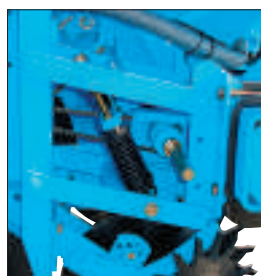
Široký a kompaktný paralelogram s nastaviteľnou pružinou.
