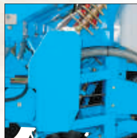
Prevodovka vzdialenosti semien s vymeniteľnými ozubenými kolesami na ľavej strane.
